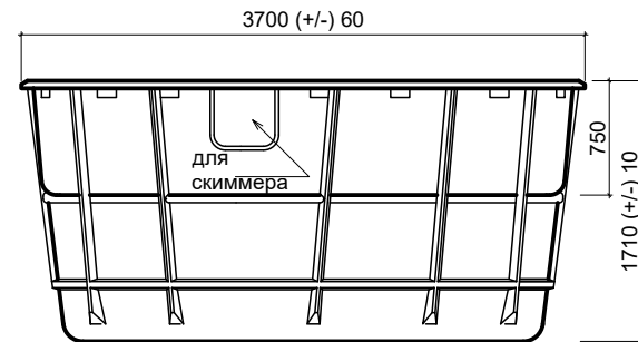
Вид А
