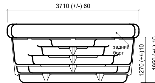
Вид А
