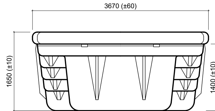
Вид В
