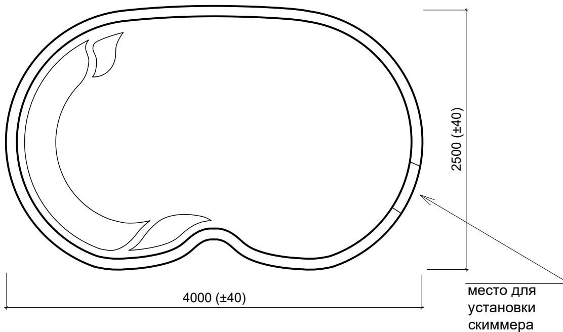
Вид А
